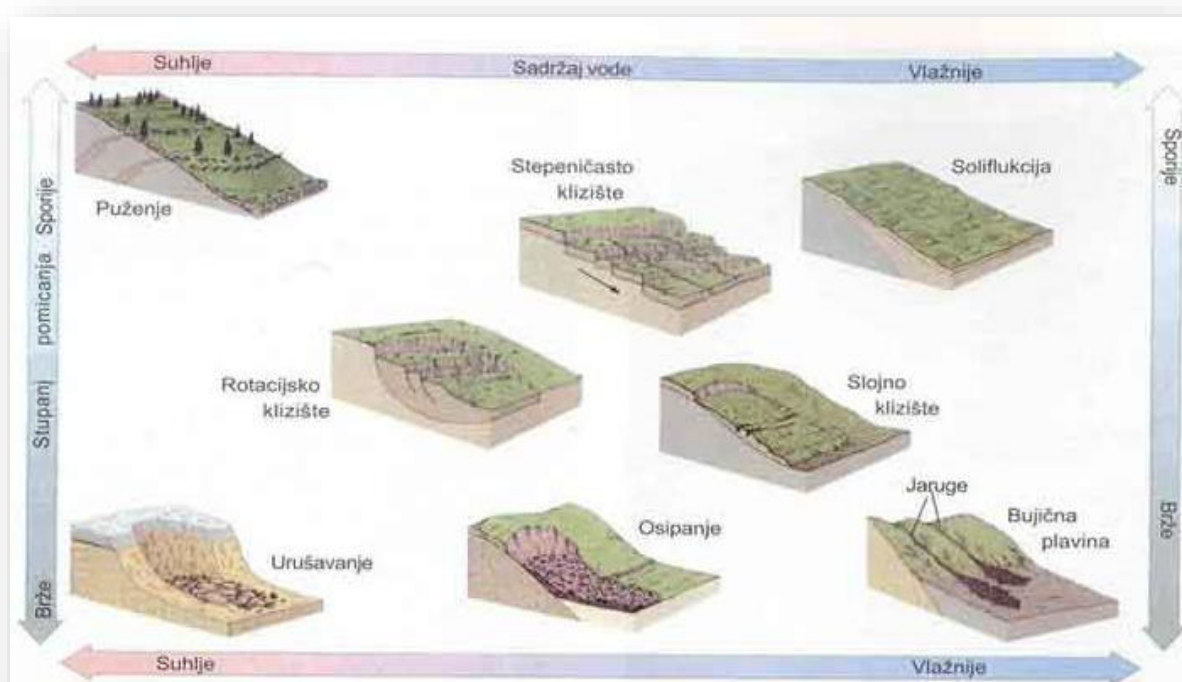
Vrste klizišta
