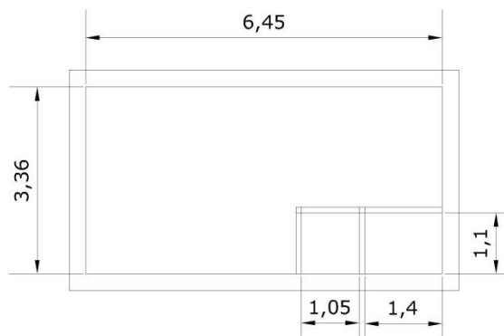
Skica-prema elab. etažiranja
